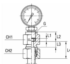
mit B3-Schneidring
