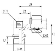
-val/-vel B4-vágógyűrűvel
