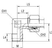
-val/-vel B4-vágógyűrűvel
