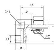
-val/-vel B3-vágógyűrűvel
