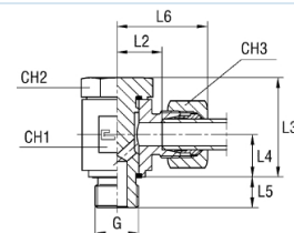
mit B3-Schneidring
