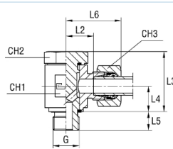
mit B4-Schneidring
