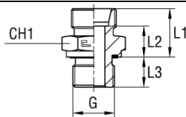
priključci sa navojem
