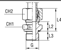
sa usečnim prstenom B3
