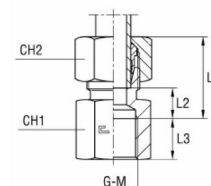
s B3 řezným kroužkem
