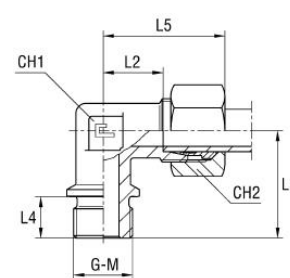
s B3 řezným kroužkem
