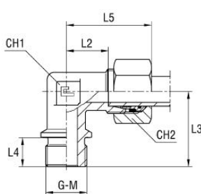
s B4 řezným kroužkem
