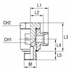
priključci sa navojem
