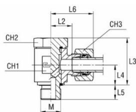
B4-es vágógyűrűvel
