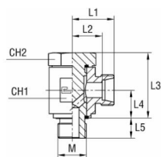
becsavarható csavarzatok
