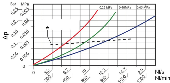
*Doporučený maximální průtok Diagram zobrazuje různé vstupní tlaky
