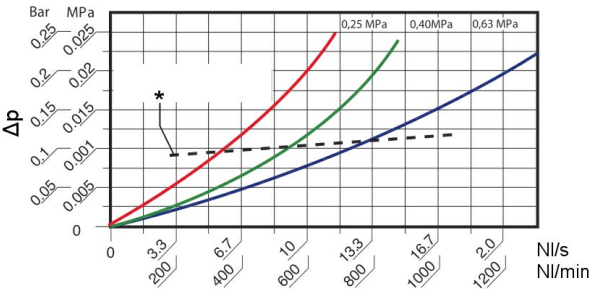
*Empfohlener maximaler Durchfluss Das Diagramm zeigt verschiedene Eingangsdrücke
