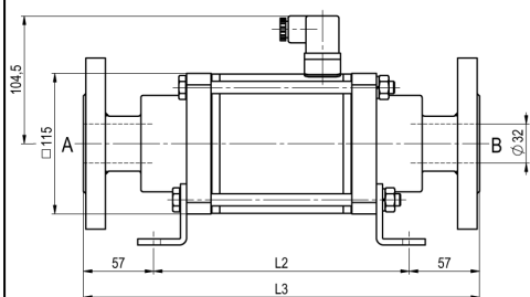
CVF-32 funkcija NO
