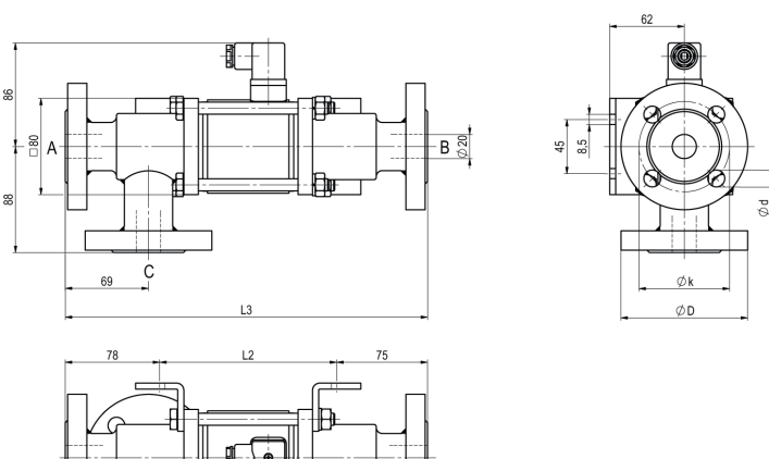
CVF3-20 funkcja NO
