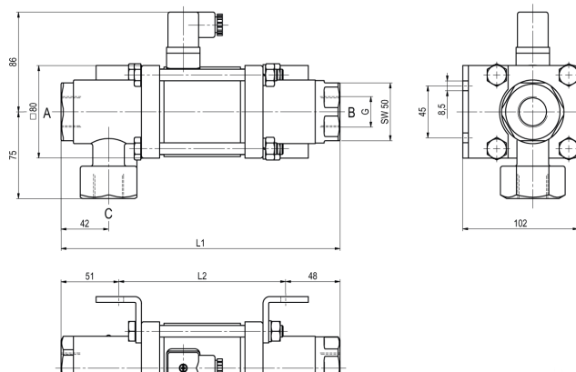
CVT3-20 funkcja NC
