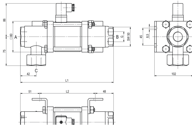
CVT3-20 function NC
