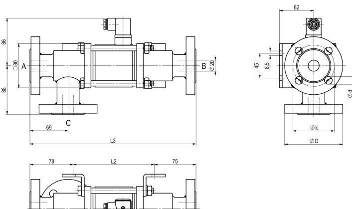
CVF3-20 function NO
