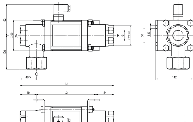
CVT3-25 Funktion NC
