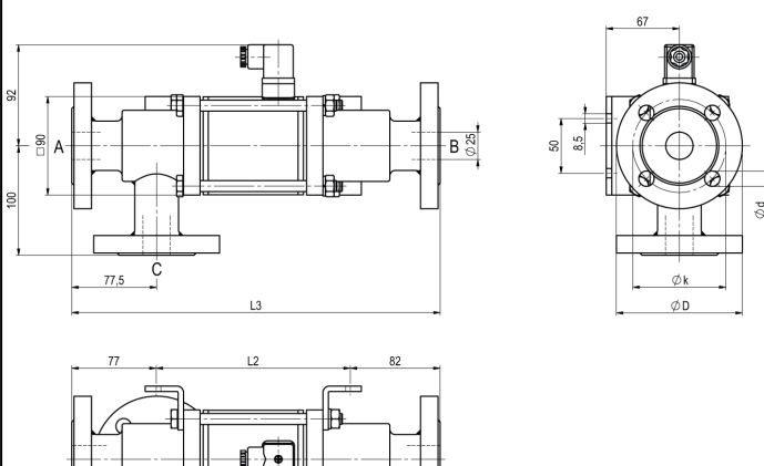
CVF3-25 Funktion NO
