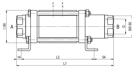
CVTE-32 funkció NC
