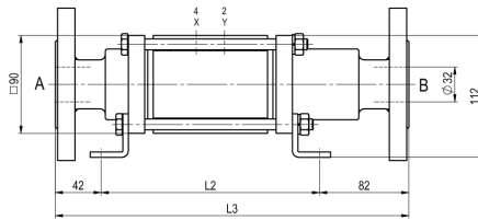
CVFE-32 funkció NO
