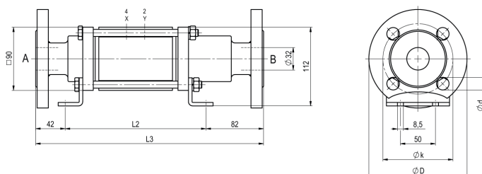
CVFE-32 funkcija NO
