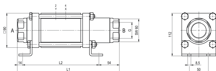
CVTE-32 funkcija NC
