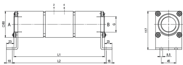
CVTV-40 function NC
