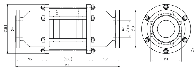
CVFV-100 Funktion NO
