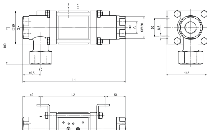
CVTE3-25 funkcja NC
