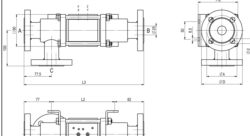
CVFE3-25 funkcja NO
