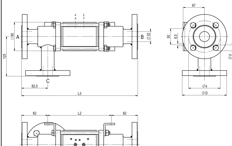
CVFE3-32 funkció NO
