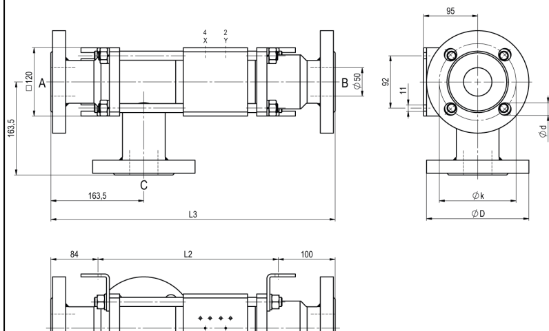
CVFE3-50 funkcija NO
