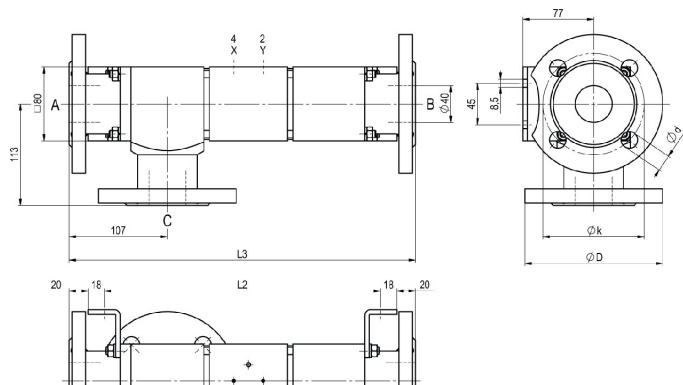
CVFV3-40 Function NO
