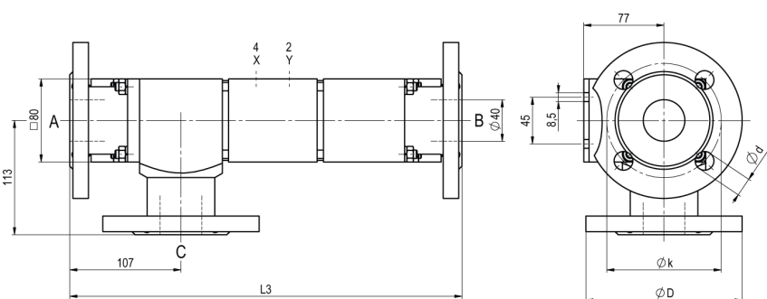
CVTV3-40 funkcija NC
