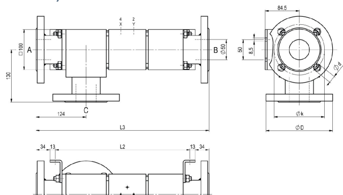
CVTV3-50 Funkcja NO
