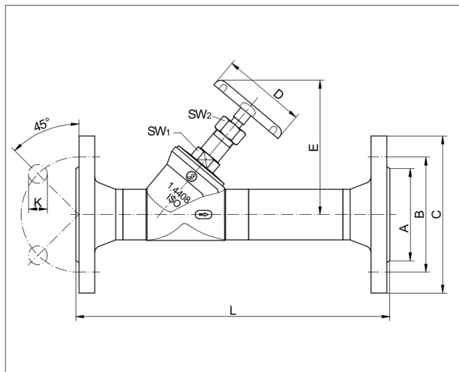
Vorschweißflansche nach DIN/ANSI
