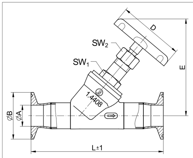
Clampstutzen nach Zoll
