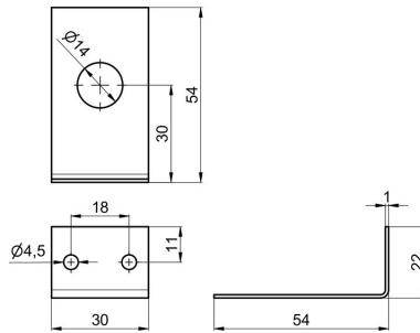
Rögzítőkonzol Típus 6403
