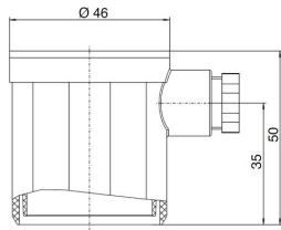
Védősapka PG-kábelátömszelencével Típus 6371 (IP54) / 6372 (IP65)
