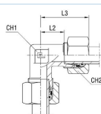
s řezným kroužkem B4
