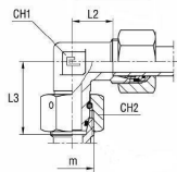
sa B4 sečnim prstenom
