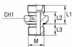
Základní těleso
