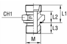
Základní těleso
