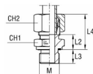
mit B3-Schneidring
