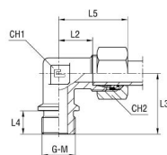
mit B4-Schneidring
