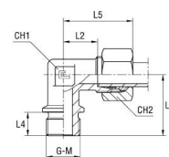
mit B3-Schneidring
