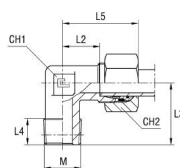
mit B4-Schneidring
