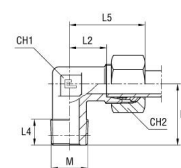
mit B3-Schneidring
