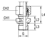
mit B4-Schneidring
