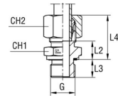
mit B3-Schneidring
