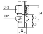
mit B3-Schneidring
