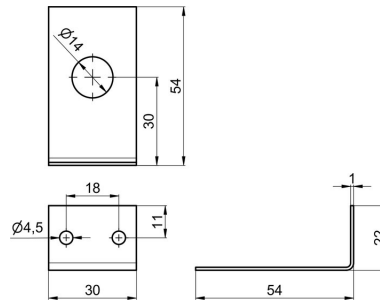
Befestigungswinkel Typ 6403
