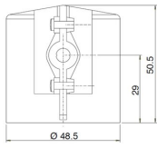
Védősapka IP44 Típus PC-PVS01-01
