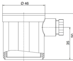
Védősapka PG-kábelátömszelencével Típus 6371 (IP54) / 6372 (IP65)
