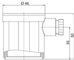
Zaštitna kapa sa PG uvodnicom Tip 6371 (IP54) / 6372 (IP65)
