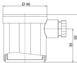
Zaščitni pokrovček s PG-kabelsko uvodnico Tip 6371 (IP54) / 6372 (IP65)
