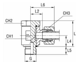
-val/-vel B3-vágógyűrűvel
