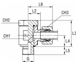
-val/-vel B4-vágógyűrűvel
