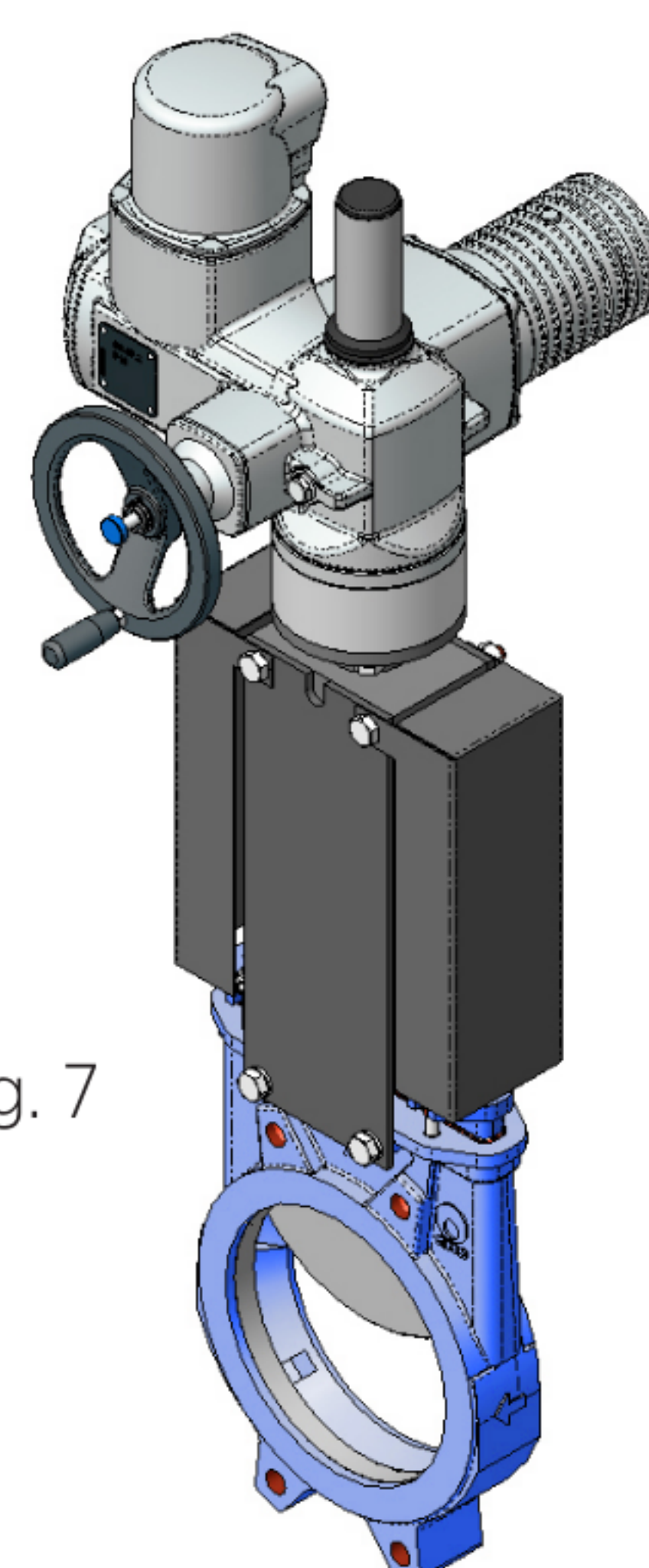
ELECTRIC-MOTOR ACTUATOR
