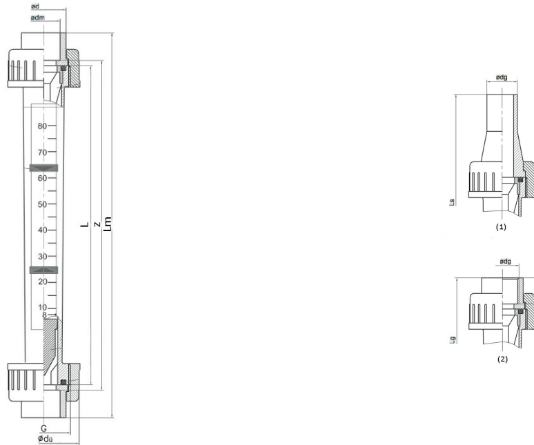
(1)...Verschraubung mit Schweißstutzen, (2)...Verschraubung mit Gewindemuffe
