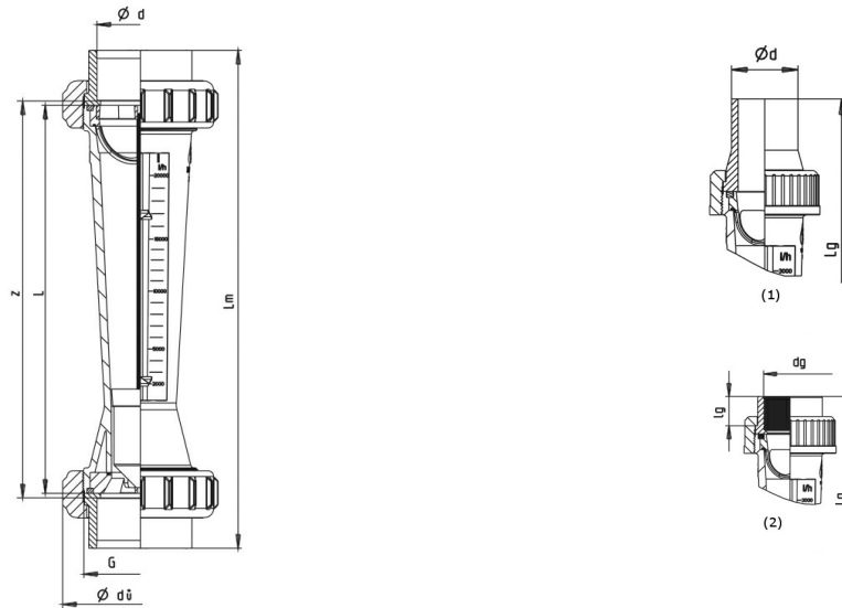
(1)...Verschraubung mit Schweißstutzen, (2)...Verschraubung mit Gewindemuffe
