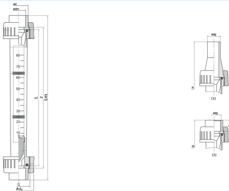
(1)...Priključak sa nastavkom za zavarivanje, (2)...Priključak sa navojnom čaurom
