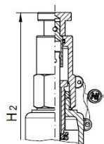
Hlava plynotěsné s odvzdušňovacím tlačítkem
