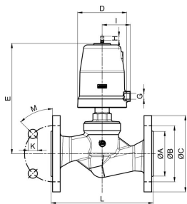
Zamykanie sprężyną, Typ SE24, SE25, SE33
