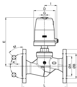
Sprężyna otwiera, Typ SE23
