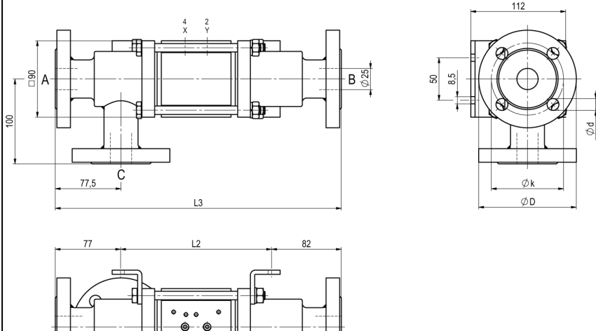
CVFE3-25 Funktion NO
