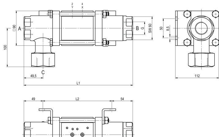
CVTE3-25 Funktion NC
