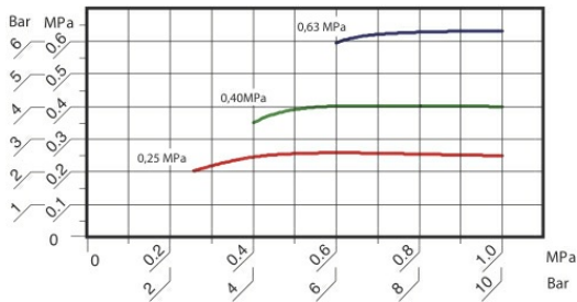
Pretok konstanten = 750NI/min horizontalna os: Vhodni tlak vertikalna os: Izhodni tlak
