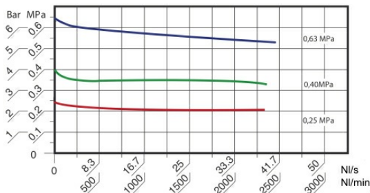
Vhodni tlak = 10bar, Pretok v normalnem stanju
