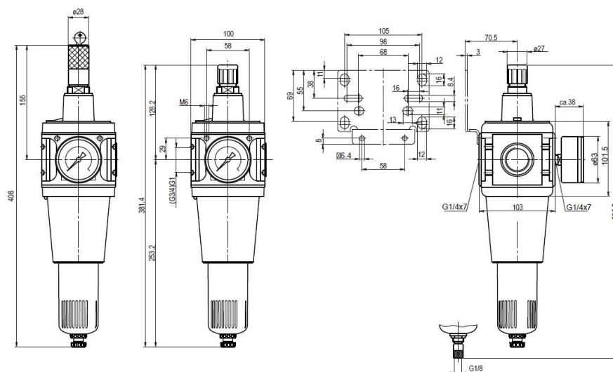
félautomata leeresztőszелеп
