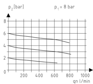
Dijagram protoka
