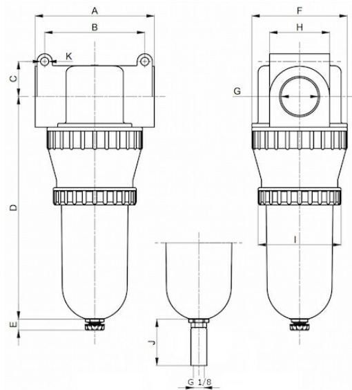
automatisches Ablassventil
