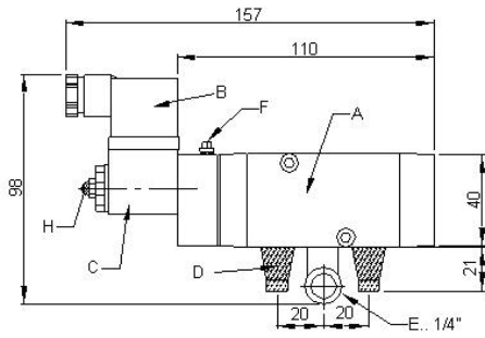
Abmessungen ABS51
