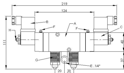
Abmessungen ABS55
