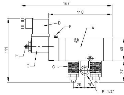
Abmessungen ABS54
