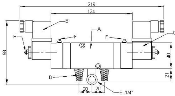
Abmessungen ABS52
