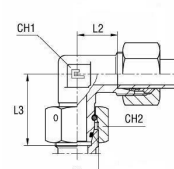
-val/-vel B3-vágógyűrűvel
