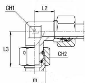
-val/-vel B4-vágógyűrűvel
